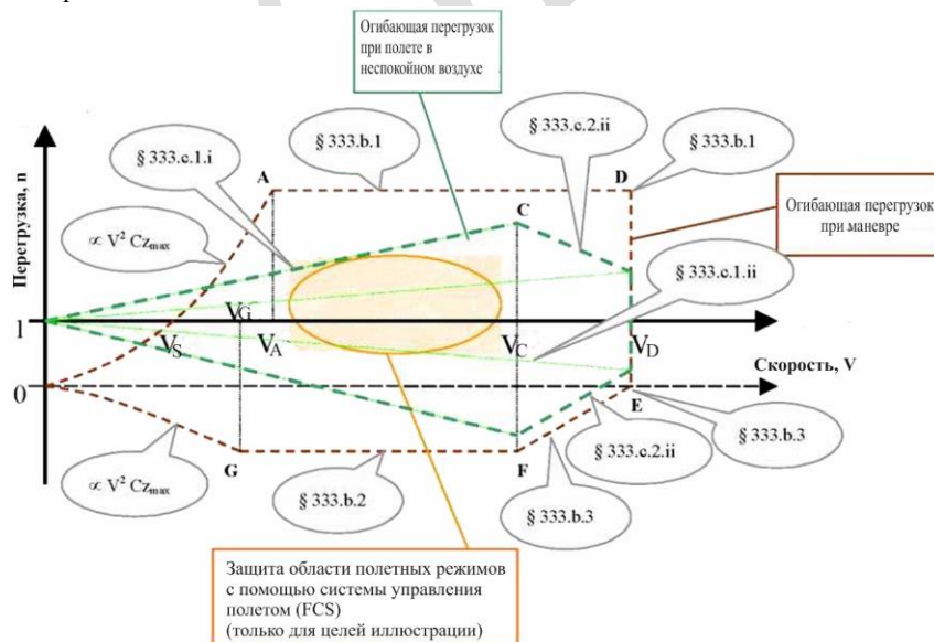
Рисунок C1. Область полетных режимов
